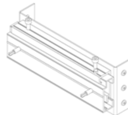
Baugruppe Agraffeneinschub für 190 mm breite Kasette
